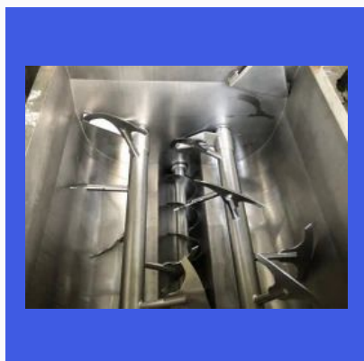
Paddle Agitator
